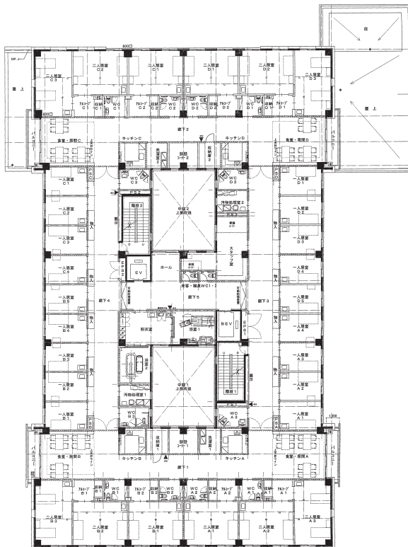
(2階平面図)
